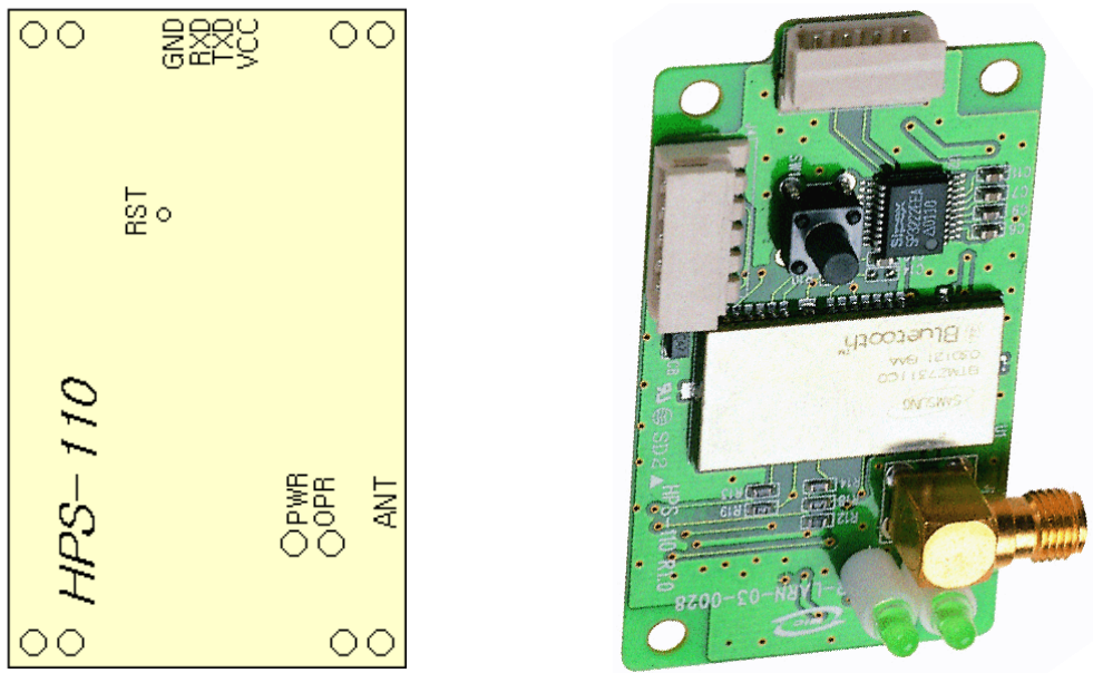
그림 2-1 제품외관정보
