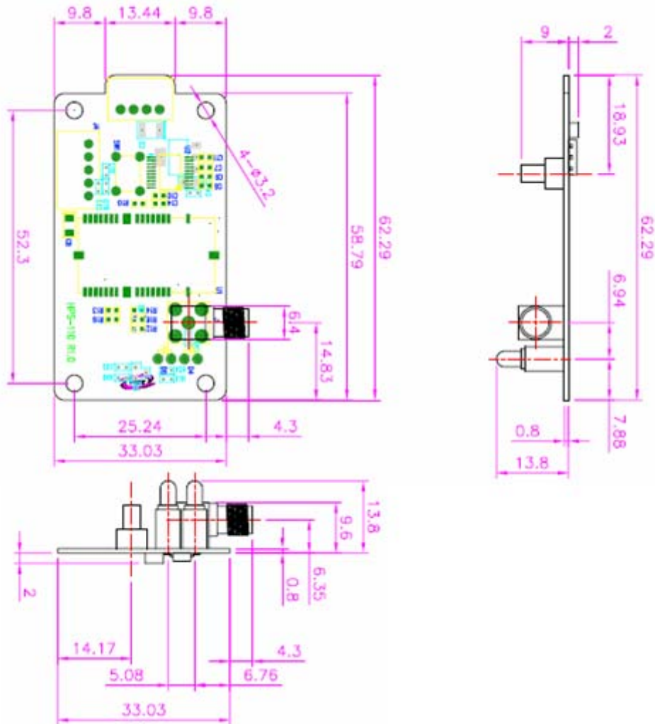
그림 2-2 PBA 크기
