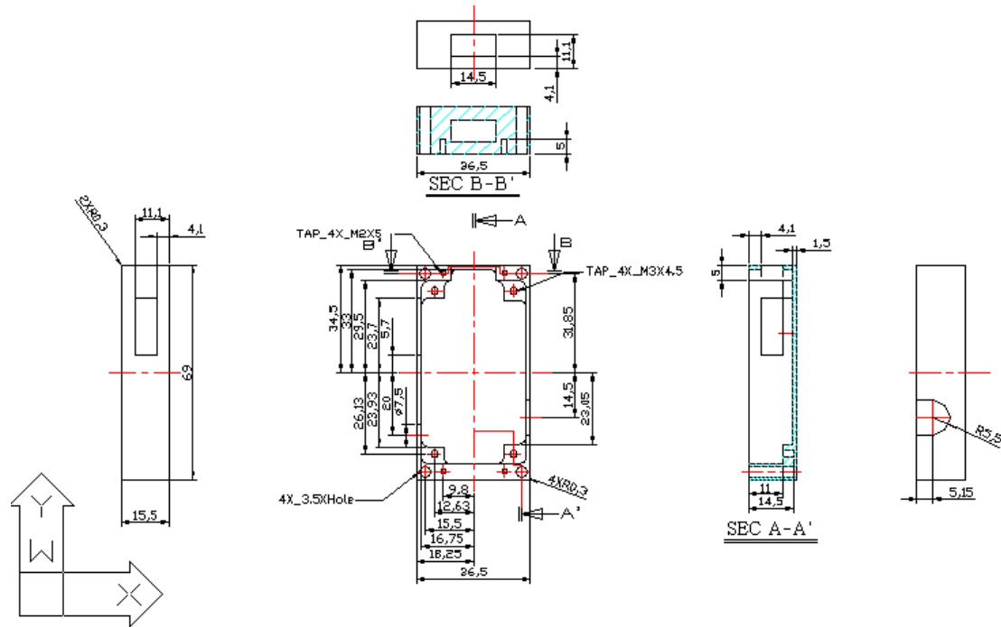
그림 2-3 합체크기
