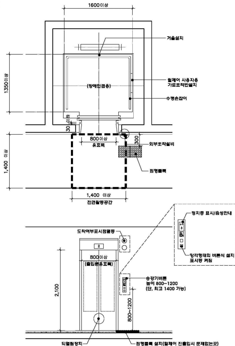
장애인용 승강기
