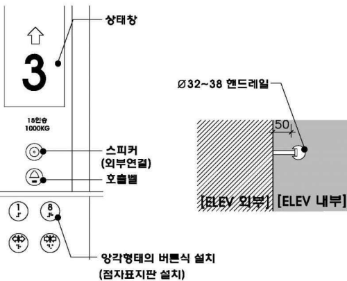
일반조작반
