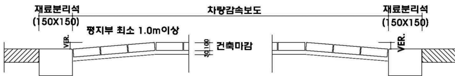
차량감속보도 횡단면도
