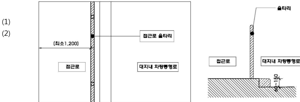
접근로 울타리
