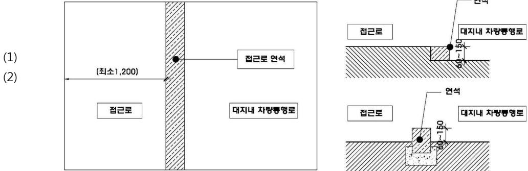
접근로 경계석
