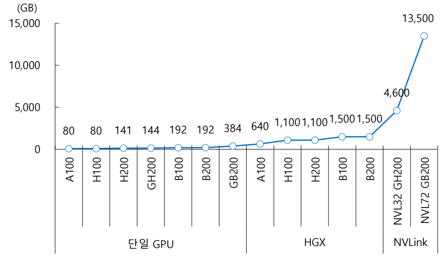
<그림> 아키텍처 진화 및 모듈, Rack 시스템 제품 등장으로 HBM 탑재 확대
