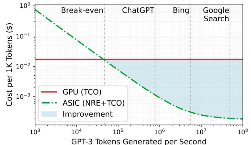
<그림> 특정 모델에 특화된 ASIC 반도체는 TCO 관점에서 합리적인 선택
