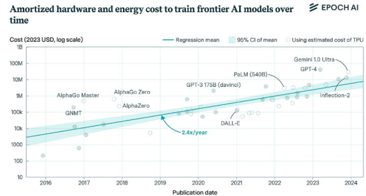
<그림> AI Scaling Law
