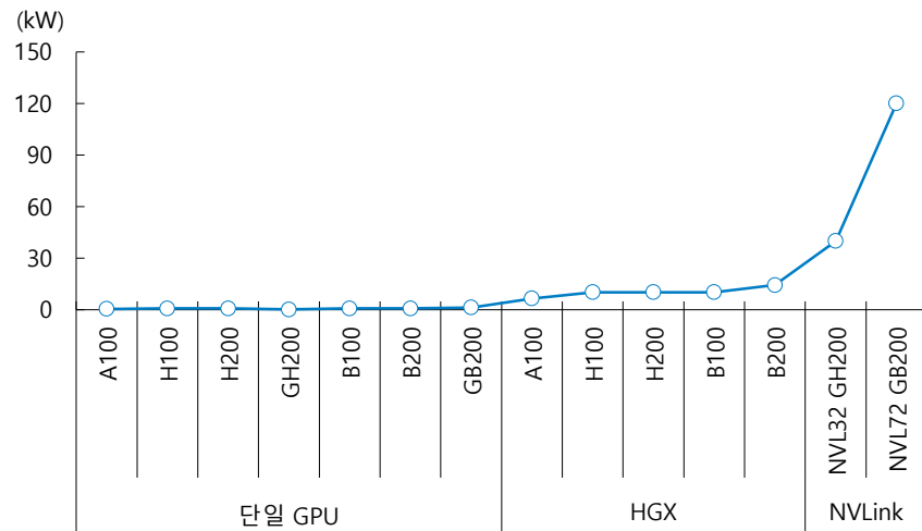
<그림> GB200 NVL72의 소비전력은 14.3kW까지 증가
