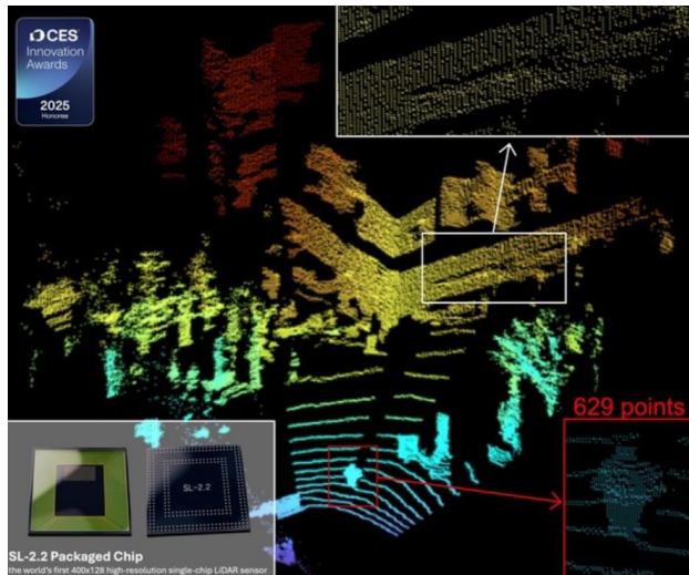
<그림> 한국 스타트업인 Solidvue의 라이다 센서 SL-2.2와 데모 이미지
