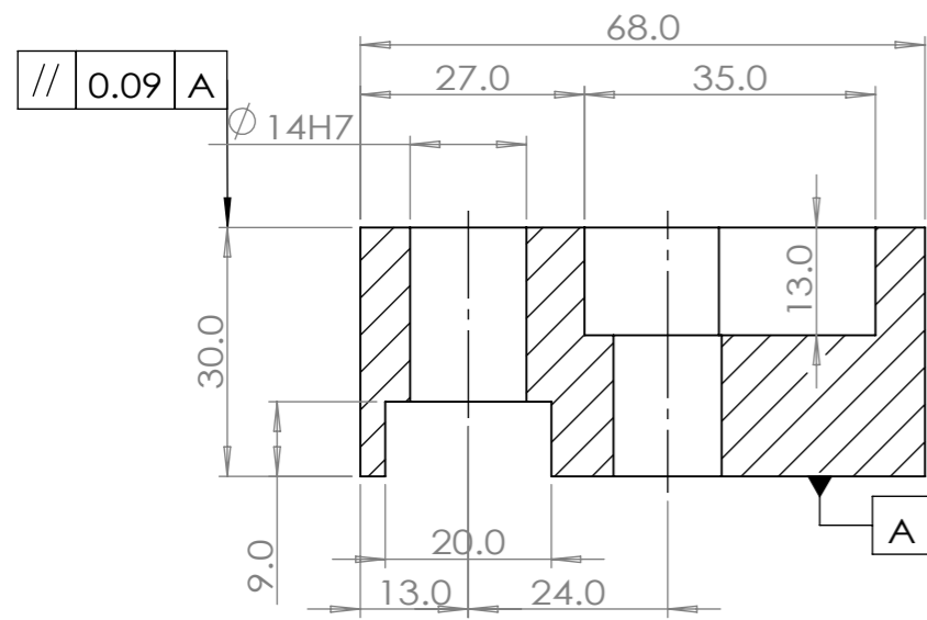
단면 A-A
