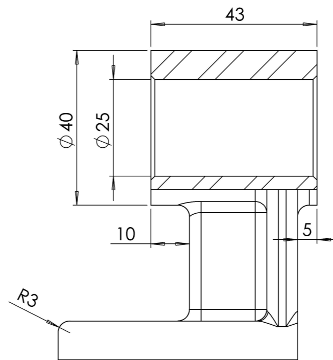
단면 A-A
