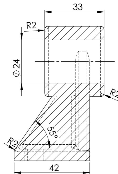
단면 E-E
