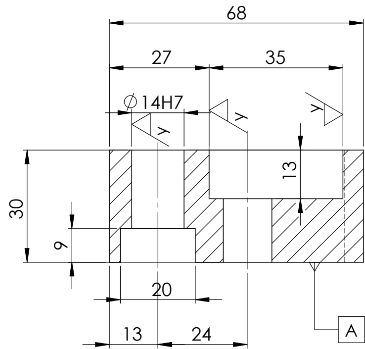
단면 A-A
