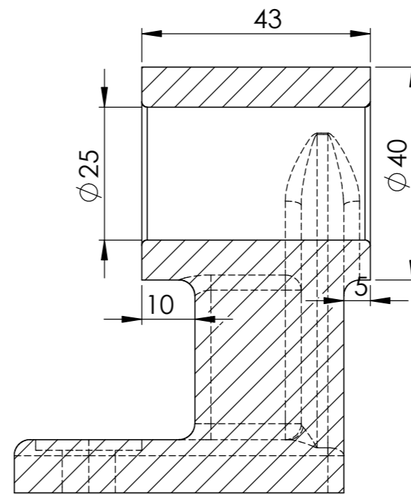
단면 D-D
