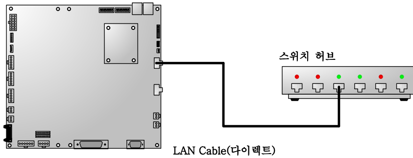
< 그림 6-9: MCM 모듈과 허브 연결 >
