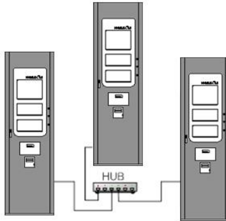
< 그림 6-7: 1대의 허브로 수신기 3개를 연결한 경우 >
