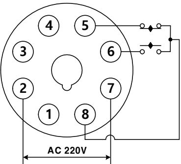
[FR 내부 결선도]
