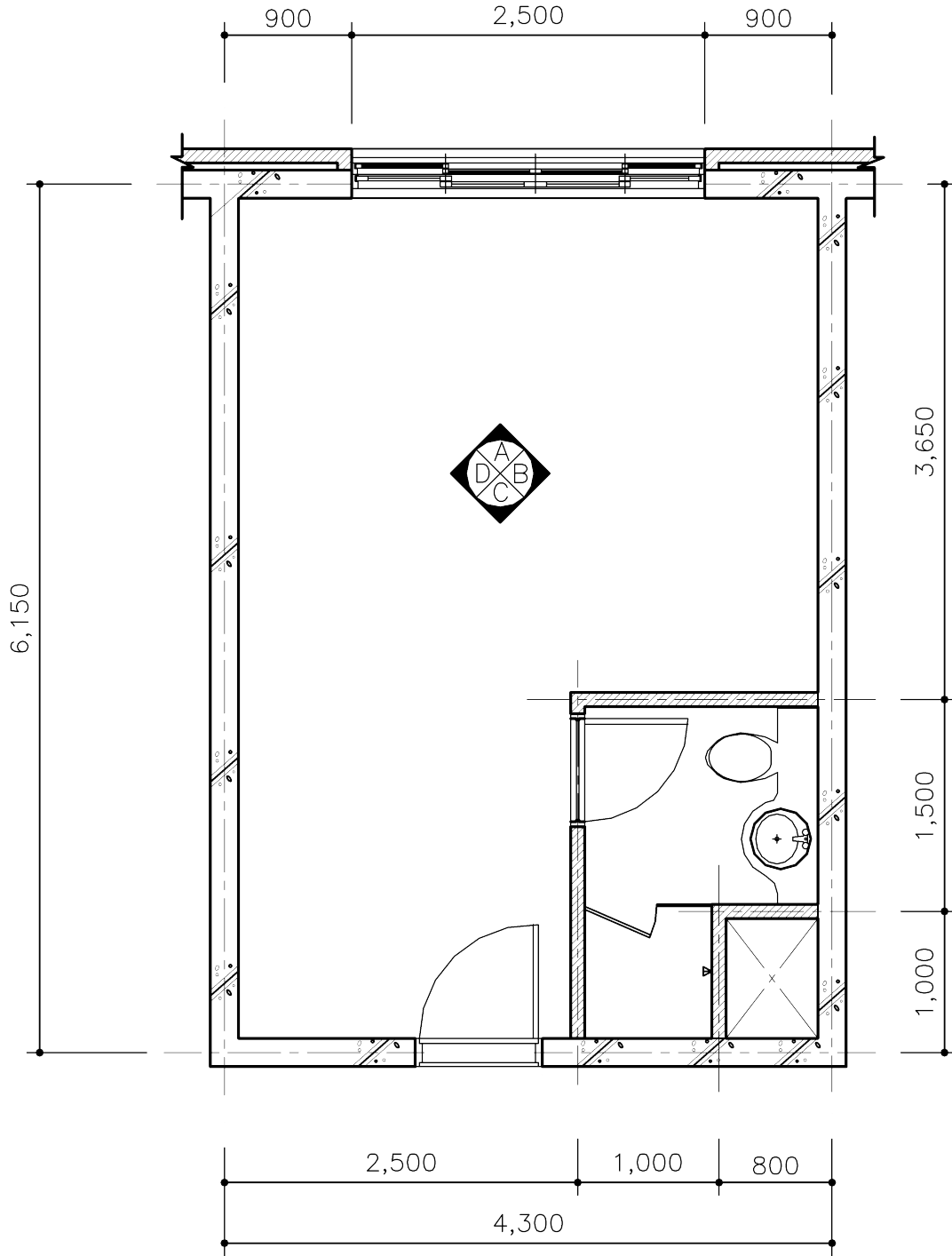
평면도
