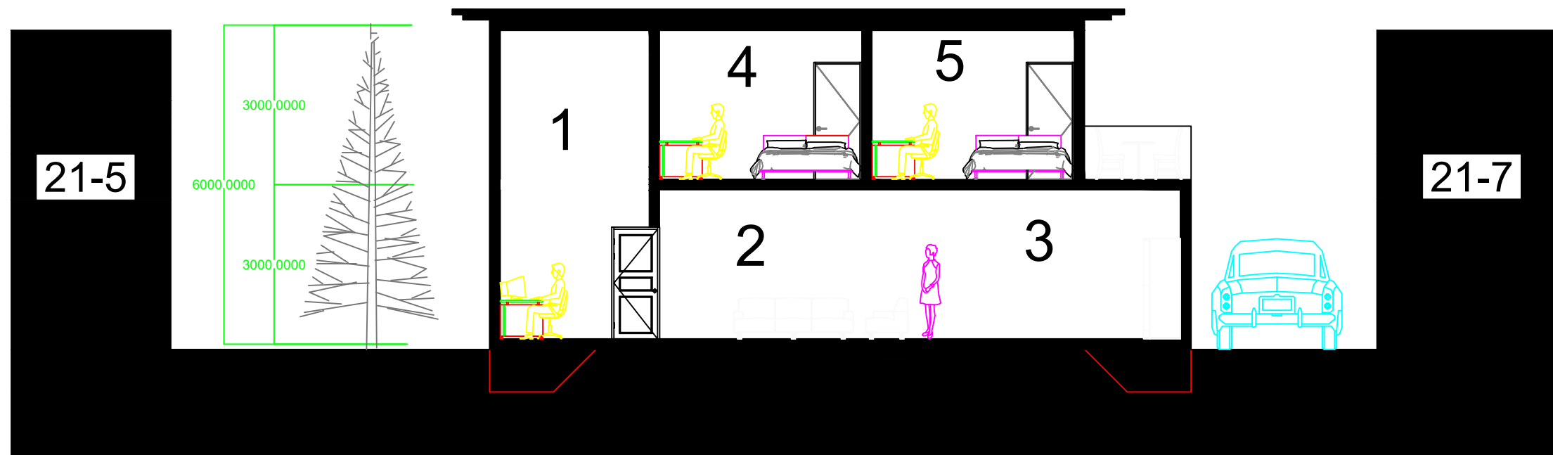
북측 단면도 축척 A3 : 1/100
