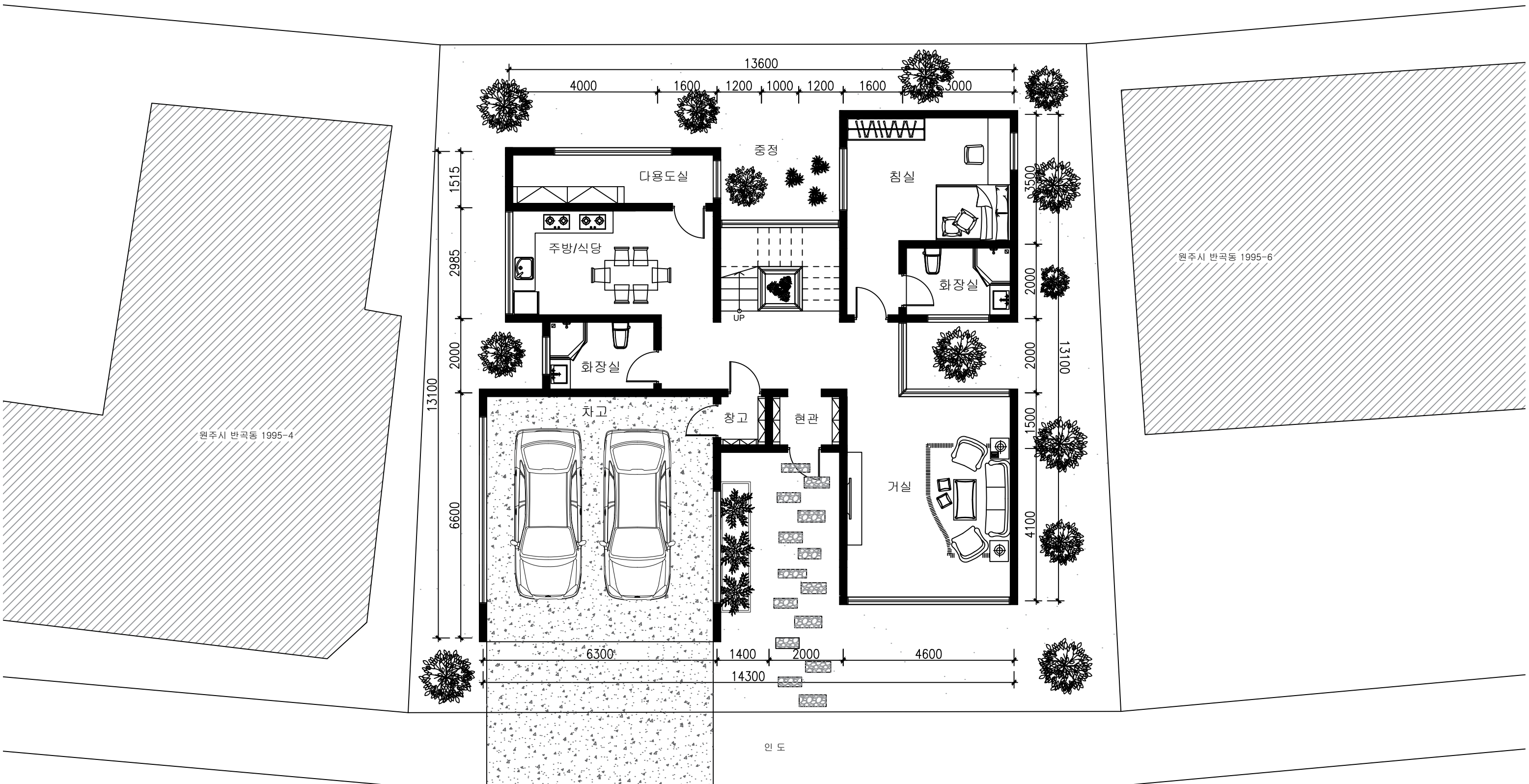
1층 평면도 축척 1:100
