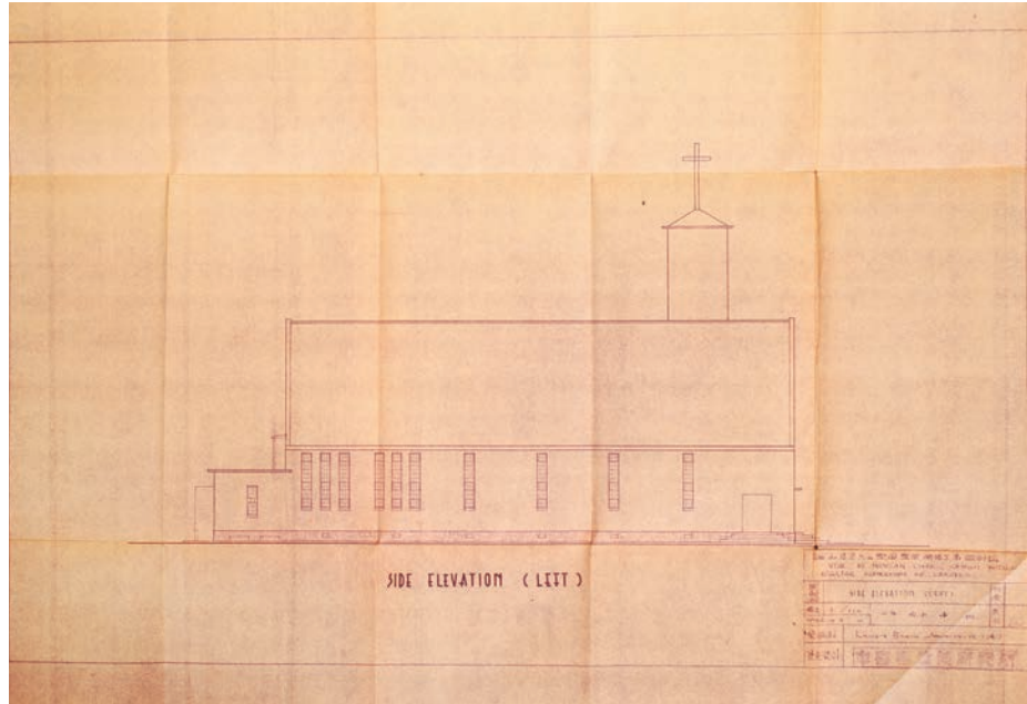
— 측면도(좌측)
