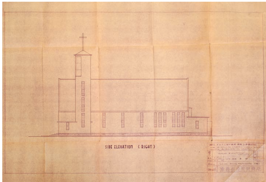
측면도(우측)
