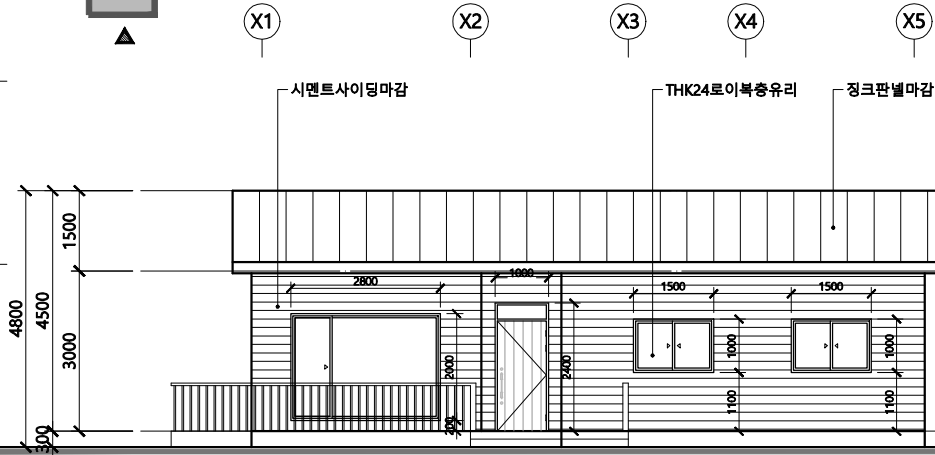
1 정면도 축척 1:100
