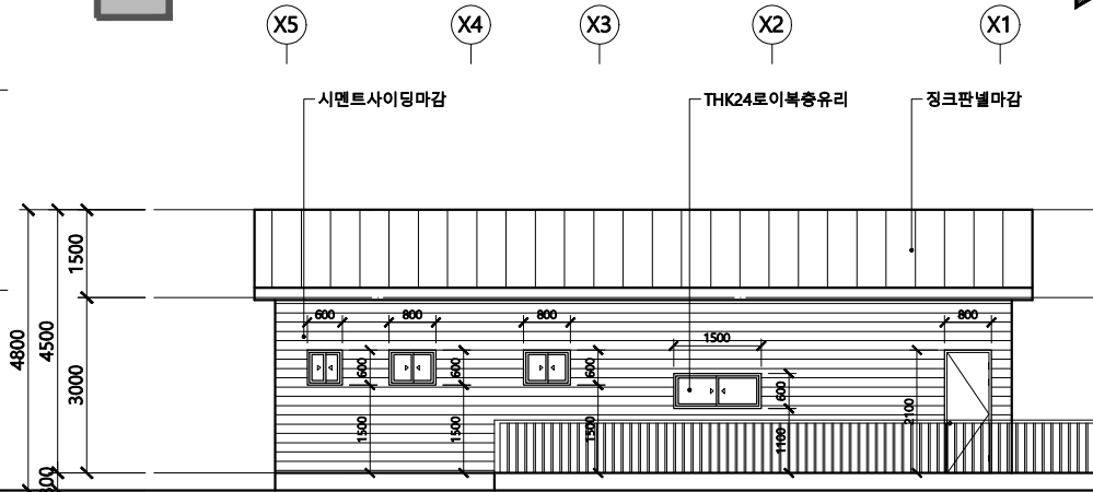
3 배면도 축척 1:100
