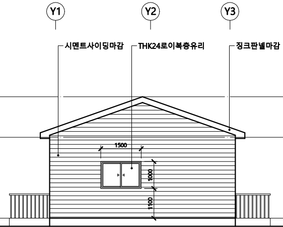
4 좌측면도 축척 1:100
