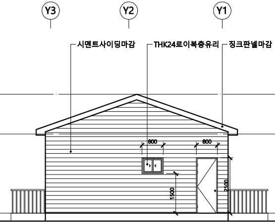
2 우측면도 축척 1:100
