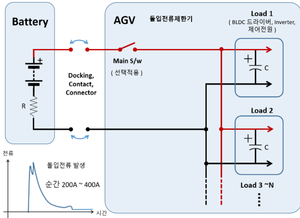
그림 1 [일반적인 계통도]
