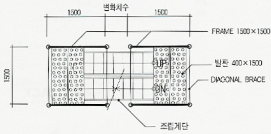
평면도
