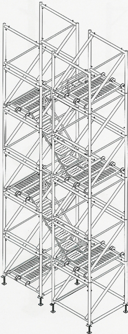
조립도
