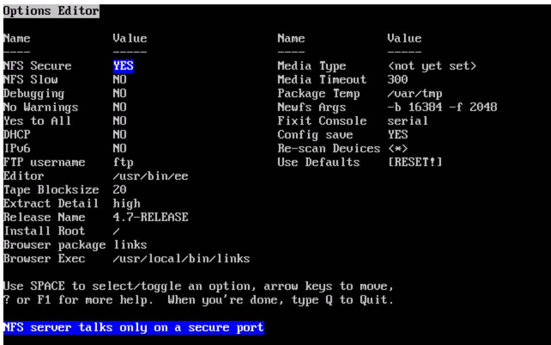
그림 2-14. Sysinstall 옵션
