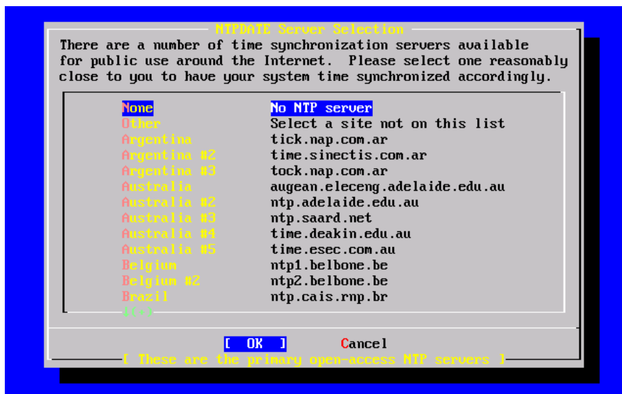
그림 2-53. Ntpdate 설정
