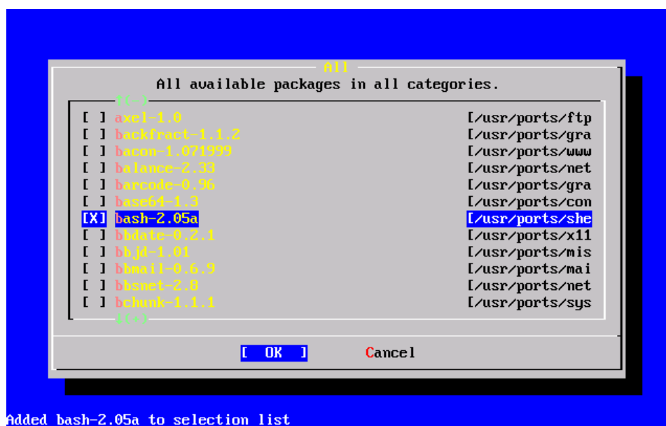
그림 2-58. 패키지 선택
